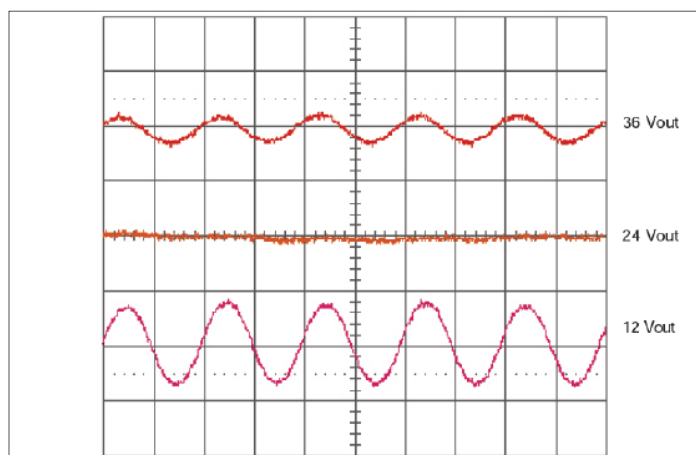
图5: 24V输入时输入端纹波电流和额定的负载电流 (500mA/div)。负载电容: 100μF 电解电容。带宽: 20MHz。见图4
