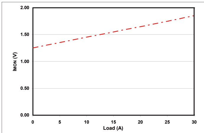
图9: 在24V输入和13.8V输出时, Imon引脚电压与负载电流的关系。负载电容: 100μF 电解电容。仅C版本。
