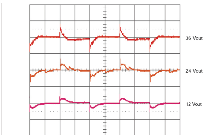
图11: 24V输入时输出电压响应; 12V、24V、36V输出电压响应 负载电流阶跃变化 (最大输出电流50%-75%-50%; di/dt = 0.1A/\mu s )。负载电容: 100μF、100mΩ钽电容。Ch1-3: Vout(2V/div):(5ms/div)
