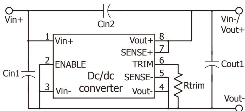
图 A “C 版本”模块电流检测及限流设定功能典型应用电路
