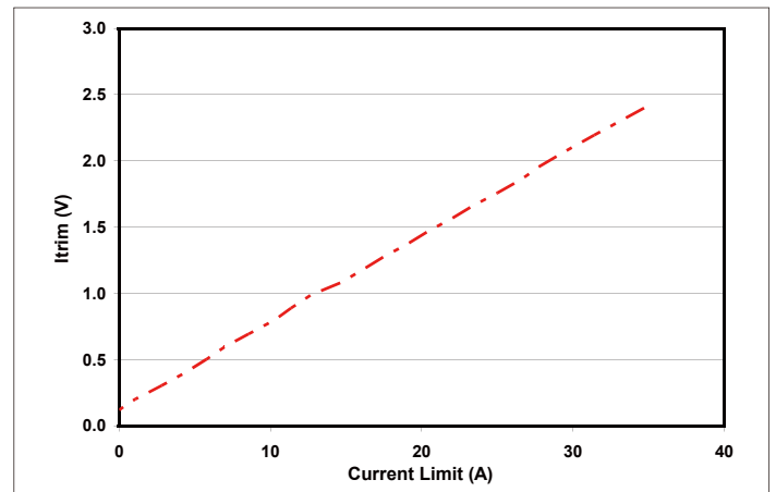
图10: 在24V输入和13.8V输出时, 限流与Itrim引脚电压的关系。负载电容: 100μF 电解电容。仅C版本。
