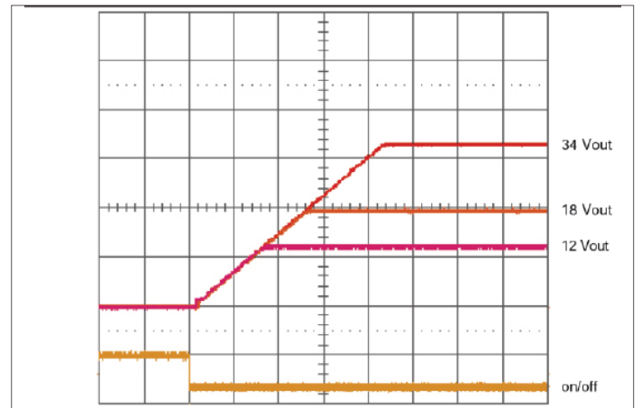
图8: 在24V输入时, 启动瞬态。零负载 (20ms/div)。ON/OFF 输入 (5V/div); Ch1-3: Vout (10V/div)
