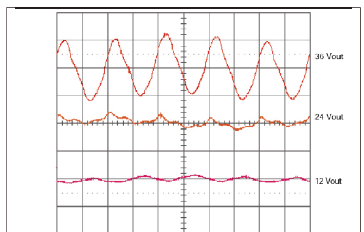
图6: 24V输入时输出电压纹波和额定的负载电流 (50mV/div)。负载电容: 100μF 电解电容。带宽: 20MHz。见图4
