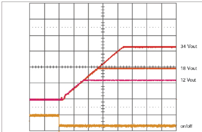
图7: 在24V输入时, 启动瞬态。满载 (20ms/div)。ON/OFF 输入 (5V/div), Ch1-3: Vout (10V/div)
