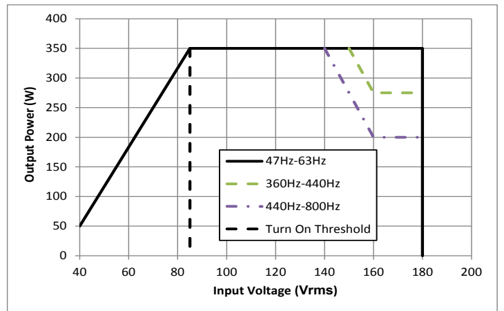
图10: 连续输出功率相对输入电压, 输出启动阈值为85Vrms
