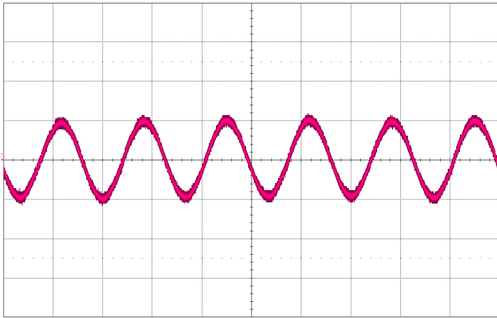
图7: 全额定功率 (115VAC, 60Hz) 时, 带400uF保持电容, 输出电压纹波, Vout (5V/div), 时基: (5ms/div)
