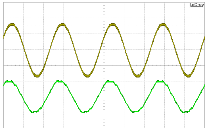
图4: 在全额定功率 (115Vrms, 400Hz) 时, 典型的输入电压和电流波形。上: Vin (100V/div), 下: Iin (5A/div), 时基: (5ms/div)
