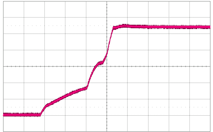
图8: 空载 (115VAC, 60Hz) 时, 带400uF保持电容, 输出电压启动波形, Vout (50V/div), 时基: (500ms/div)
