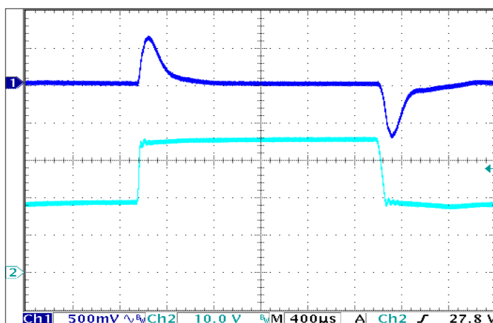
图6: 输出电压响应输入电压阶跃变化 (标称到最大输入电压) 负载电容: 100\mu\text{F} 电解输出电容。通道1: Vout (500mV/div), 通道2: Vin (10V/div)
