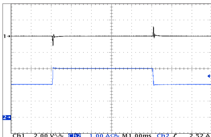
图5: 输出电压响应负载电流阶跃变化 (50%-75%-50% Iout(max)); di/dt = 0.08 \text{ A}/\mu\text{s} 。负载电容: 1\mu\text{F} 陶瓷电容。通道1: Vout (2V/div), 通道2: Iout (1A/div)
