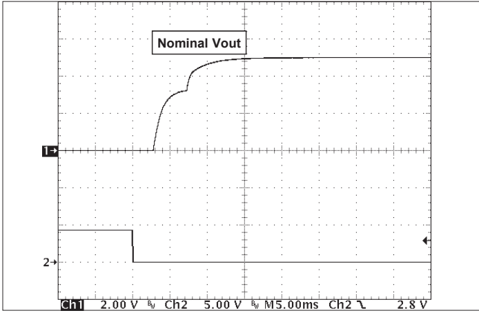
通用图 1: 典型启动波形, 输入电压提前接入, 通道 2 为 ON/OFF 引脚电压。
