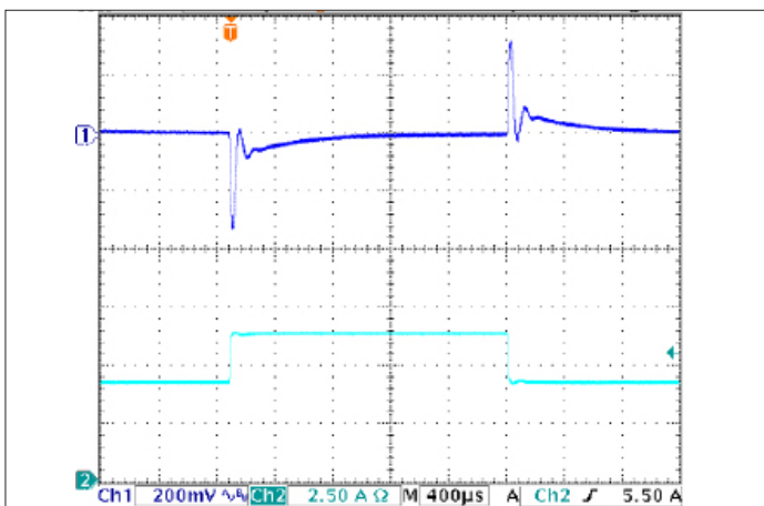
图5: 输出电压响应负载电流阶跃变化 (50%-75%-50% of Iout(max); dI/dt = 0.1 \text{ A}/\mu\text{s} )。负载电容: 1μF 陶瓷电容和 15μF 钽电容。通道1: Vout, 通道2: Iout (5A/div.)
