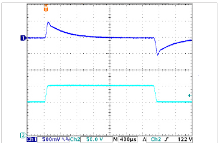
图6: 输出电压响应输入电压阶跃变化（1V / \mu\text{s} ）。负载电容：1 \mu\text{F} 陶瓷电容和15 \mu\text{F} 钽电容。通道1: Vout, 通道2: Vin。
