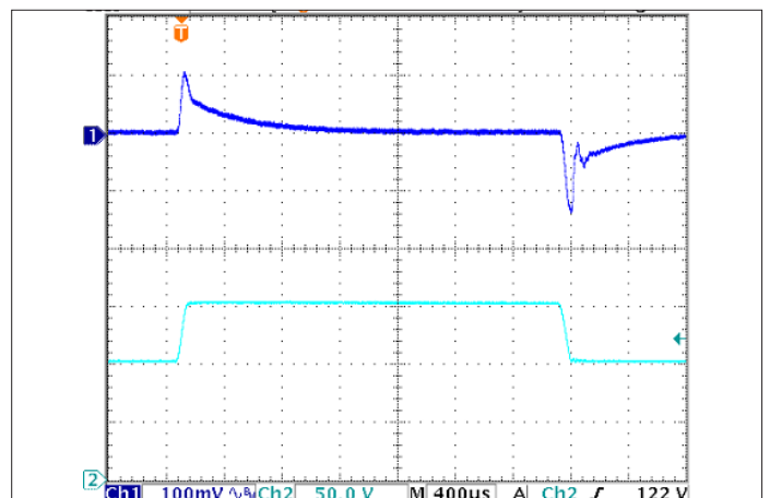
图6: 输出电压响应输入电压阶跃变化 ( 1\text{V}/\mu\text{s} )。负载电容: 1μF 陶瓷电容和 15μF 钽电容。通道1: Vout, 通道2: Vin。
