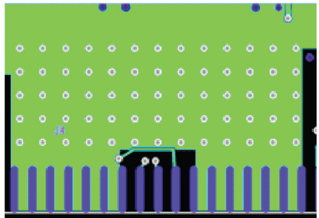
图 B：测试板上转换器周围散热孔布局图
