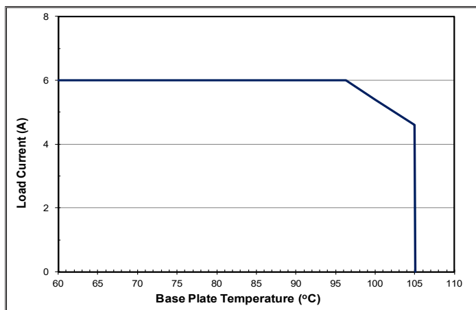
图3: 全密封转换器 (带传导散热) 最大输出功率降额相对基板温度 (标称输入电压)
