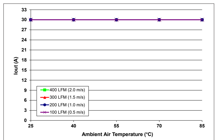
图4: 全密封转换器（1/2"散热器）最大输出电流降额相对气流速率为100 LFM至400 LFM的环境空气温度。空气从引脚3到引脚1穿过转换器（标称输入电压）
