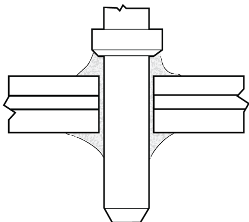
图 A：正确焊接的引脚点示例
