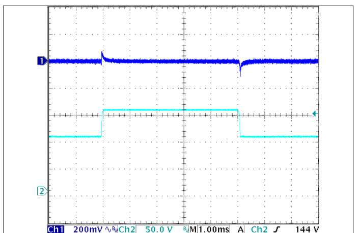
图6: 输出电压响应输入电压阶跃变化 ( 1V/\mu s )。负载电容: 1\mu F 陶瓷电容和 15\mu F 钽电容。通道1: Vout, 通道2: Vin。
