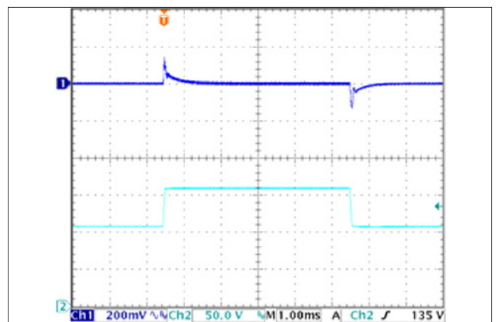
图6: 输出电压响应输入电压阶跃变化 (1V/μs)。负载电容: 1μF 陶瓷电容和 15μF 钽电容。通道1: Vout, 通道2: Vin。
