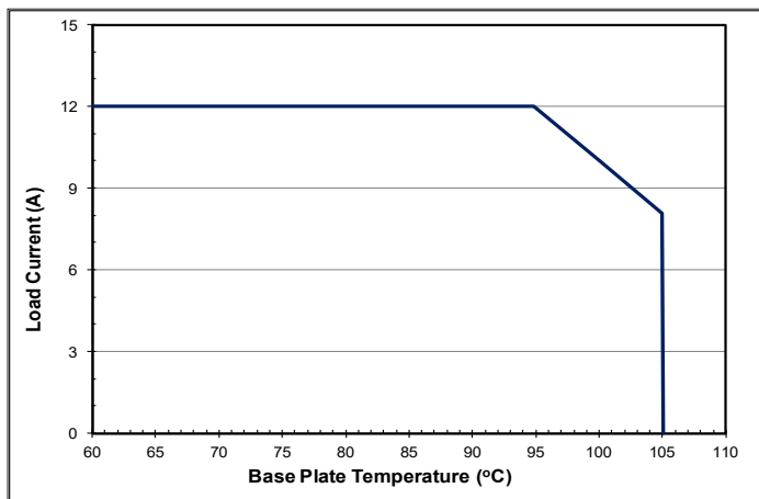
图3: 全密封转换器 (带传导散热) 最大输出功率降额相对基板温度 (标称输入电压)
