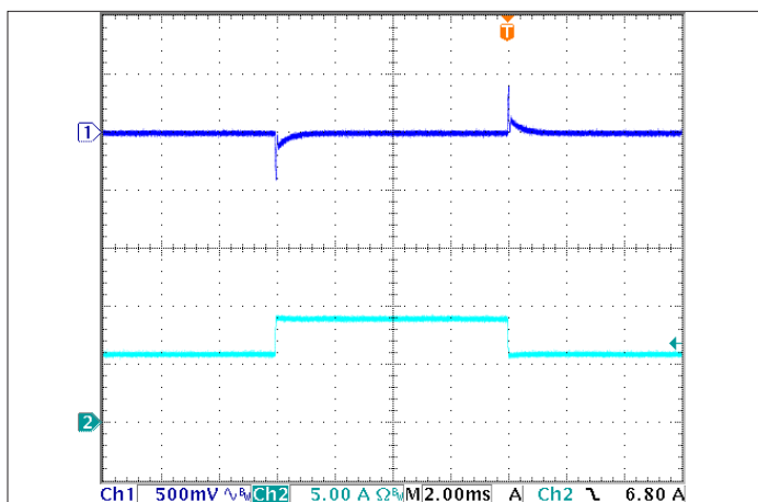
图5: 输出电压响应负载电流阶跃变化 (50%-75%-50% of Iout(max); di/dt = 0.1 A/μs)。负载电容: 1μF 陶瓷电容和 15μF 钽电容。通道1: Vout, 通道2: Iout (5A/div。)
