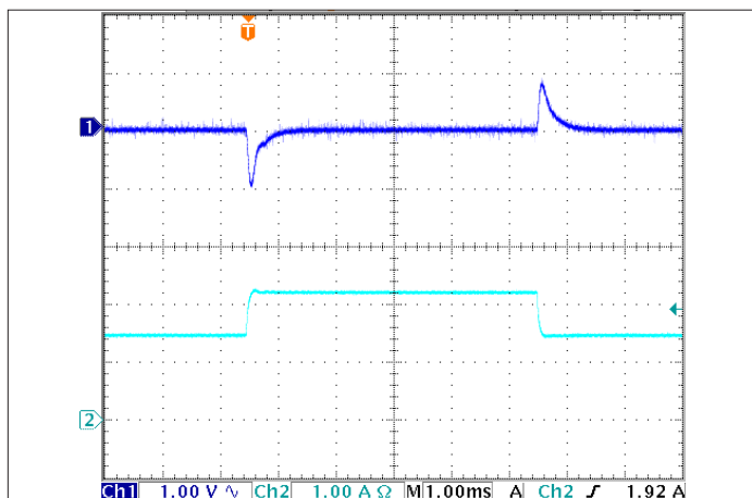
图5: 输出电压响应负载电流阶跃变化 (50%-75%-50% of Iout(max); di/dt = 0.1 \text{ A} / \mu\text{s} )。负载电容: 1\mu\text{F} 陶瓷电容和 15\mu\text{F} 钽电容。通道1: Vout, 通道2: Iout (5A/div.)
