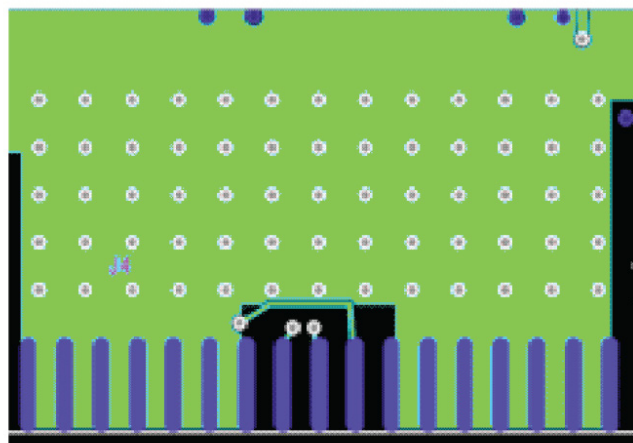
图 B：测试板上转换器周围散热孔布局图
