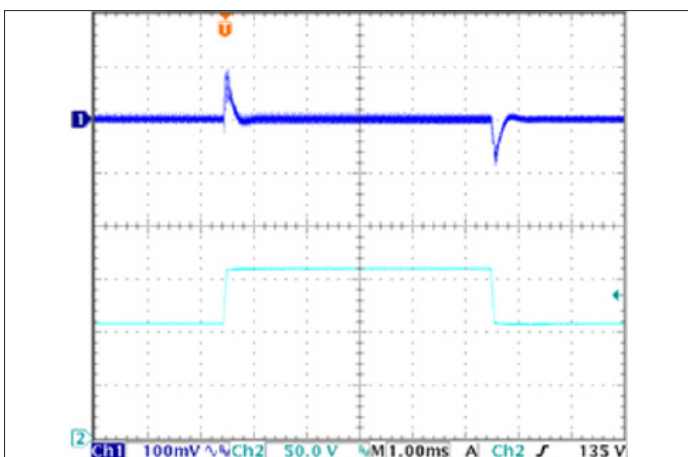
图6: 输出电压响应输入电压阶跃变化 (1V / μs)。负载电容: 1μF 陶瓷电容和 15μF 钽电容。通道1: Vout, 通道2: Vin。
