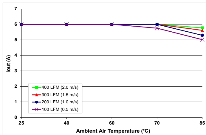
图4: 全密封转换器 (1/2"散热器) 最大输出电流降额相对气流速率为100 LFM至400 LFM的环境空气温度。空气从引脚3到引脚1穿过转换器 (标称输入电压)
