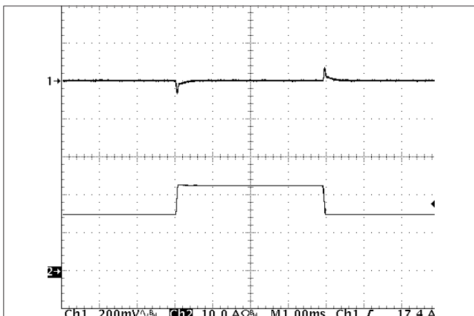
图5: 输出电压响应负载电流阶跃变化 (50%-75%-50% of Iout(max); di/dt = 0.1 A/\mu s )。负载电容: 1\mu F 陶瓷电容和 15\mu F 钽电容。通道1: Vout, 通道2: Iout (5A/div。)
