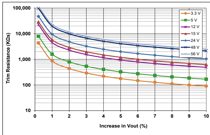
通用图 3: 3.3V 到 56V 输出电压上调阻值曲线
