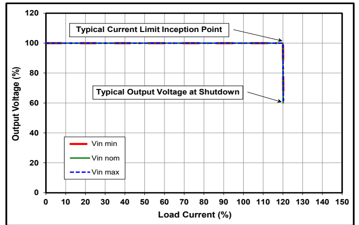
通用图 2: 输出电压相对负载电流显示典型限流曲线和转换器关断点。
