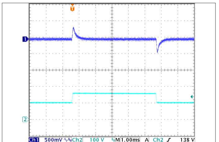
图6: 输出电压响应输入电压阶跃变化 ( 1\text{V} / \mu\text{s} )。负载电容: 1\mu\text{F} 陶瓷电容和 15\mu\text{F} 钽电容。通道1: Vout, 通道2: Vin
