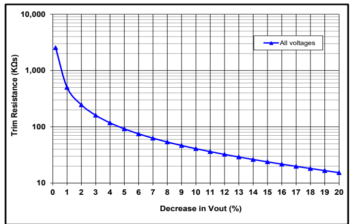
通用图 4: 输出电压下调阻值曲线
