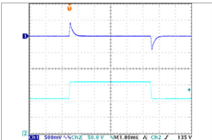
图6: 输出电压响应输入电压阶跃变化 (1V/ \mu s )。负载电容: 1 \mu F 陶瓷电容和 15 \mu F 钽电容。通道1: Vout, 通道2: Vin。
